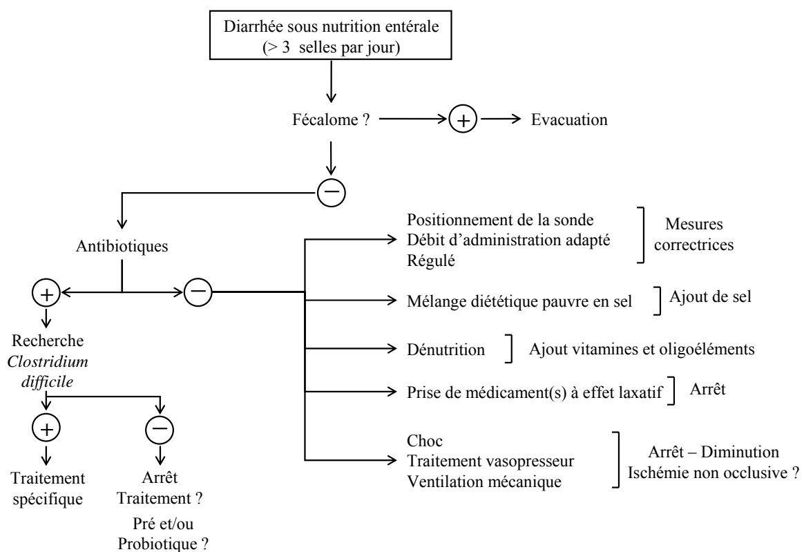
Figure 2. Approche diagnostique et thérapeutique de la diarrhée en réanimation.
